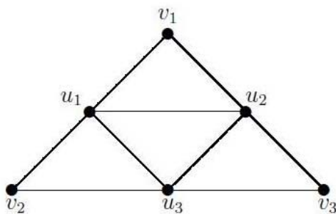
Fig. 2. Hajos graph
